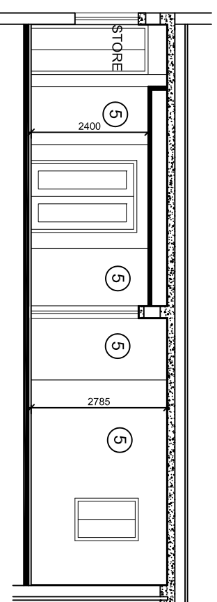
SECTION D-D
